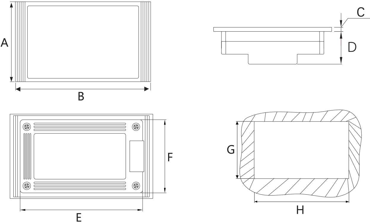
Установочные размеры выносных панелей управления W2/W3
