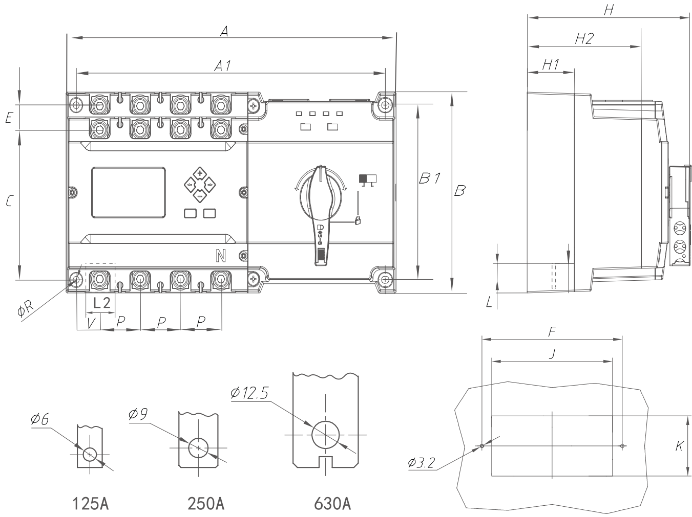
Размер выреза для установки панели контроллера на дверцу шкафа
