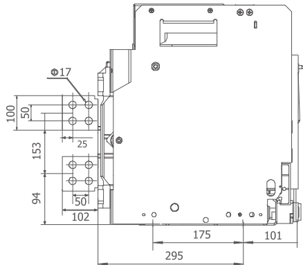
6300A, 7500A Вертикальное подключение
