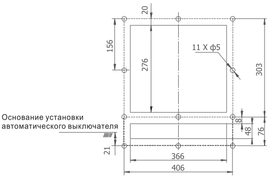
Размеры проема в дверце шкафа
