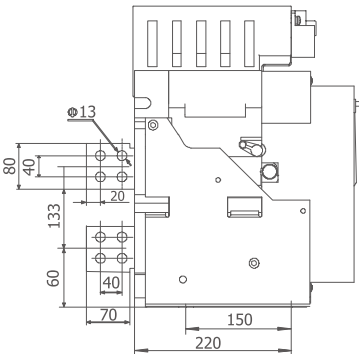
4000А, 5000А Вертикальное подключение
