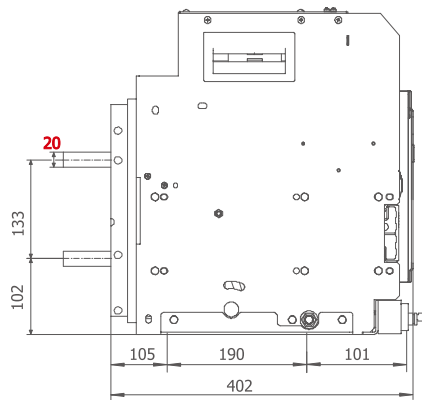
4000A, 5000A Горизонтальное подключение
