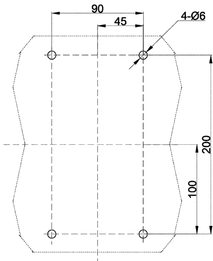
4P: Монтаж на панели
