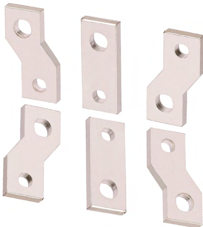
Габаритные размеры дополнительных шин для переднего подключения
